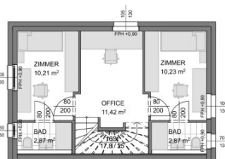
Obergeschoss
