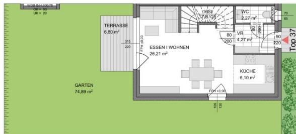
Erdgeschoss
