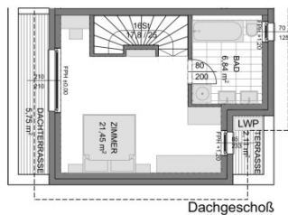
Dachgeschoss
