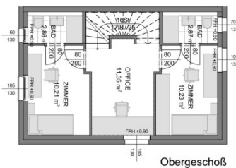
Obergeschoss
