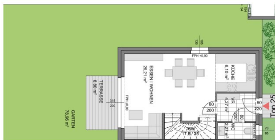
Erdgeschoss
