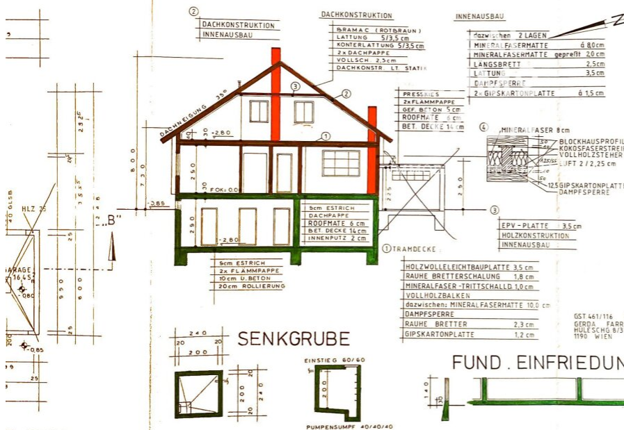
SCHNITT „A“-„B“
