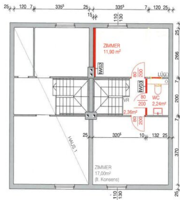
Grundriss Dachgeschoss 1:100
