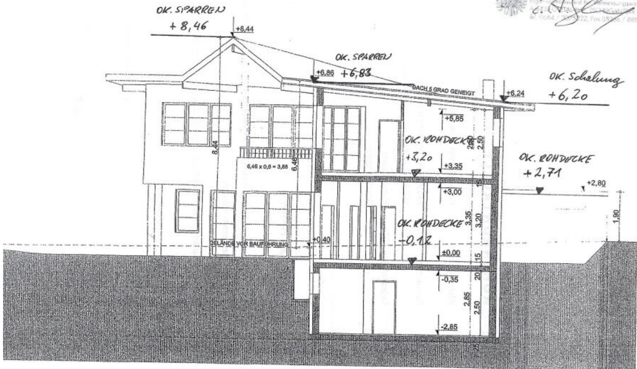
SNITT A-A
