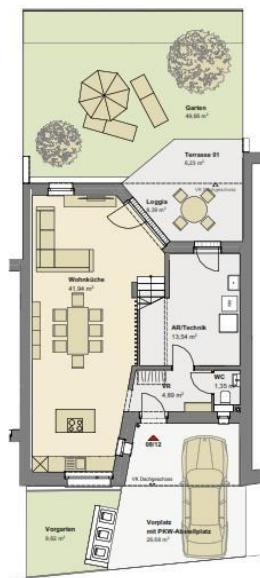
ERDGESCHOSS
