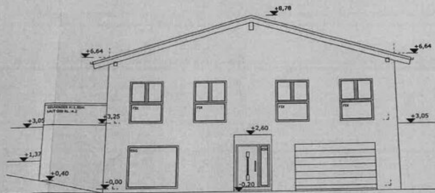
SUED-ANSICHT 1:100
