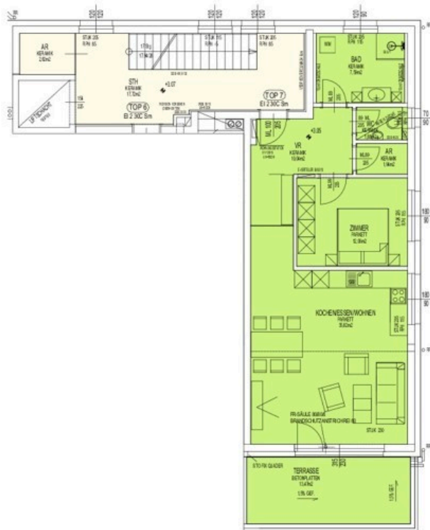
Grundriss 0 1 2 3 4 5m
