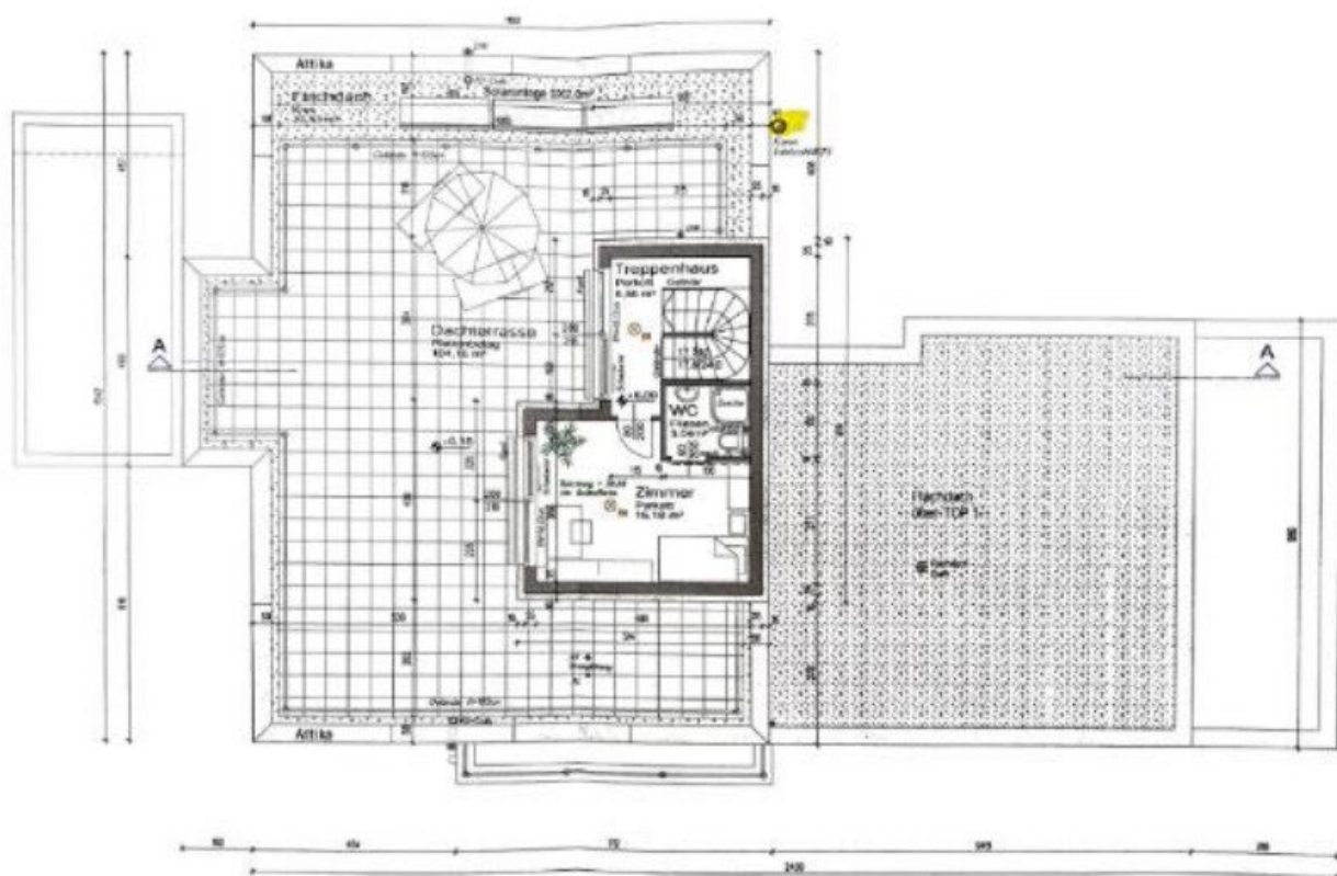
2. OBERGESCHOSS
