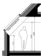
Schnitt 2
