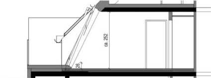
Schnitt 48.A
