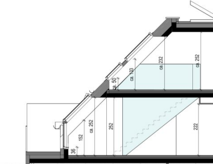
Schnitt 48.B
