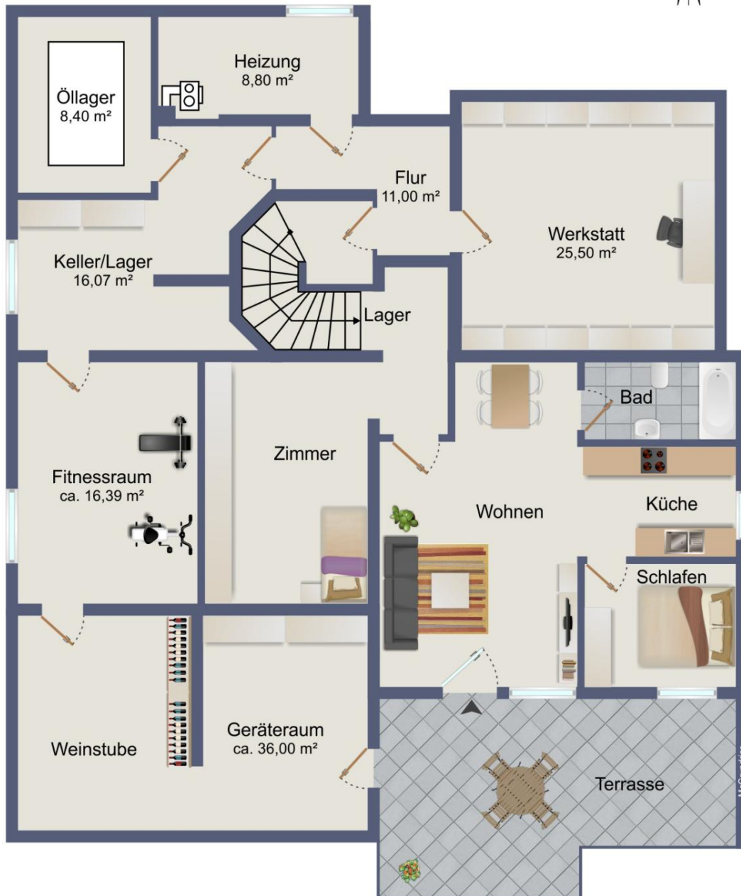
Kellergeschoss
