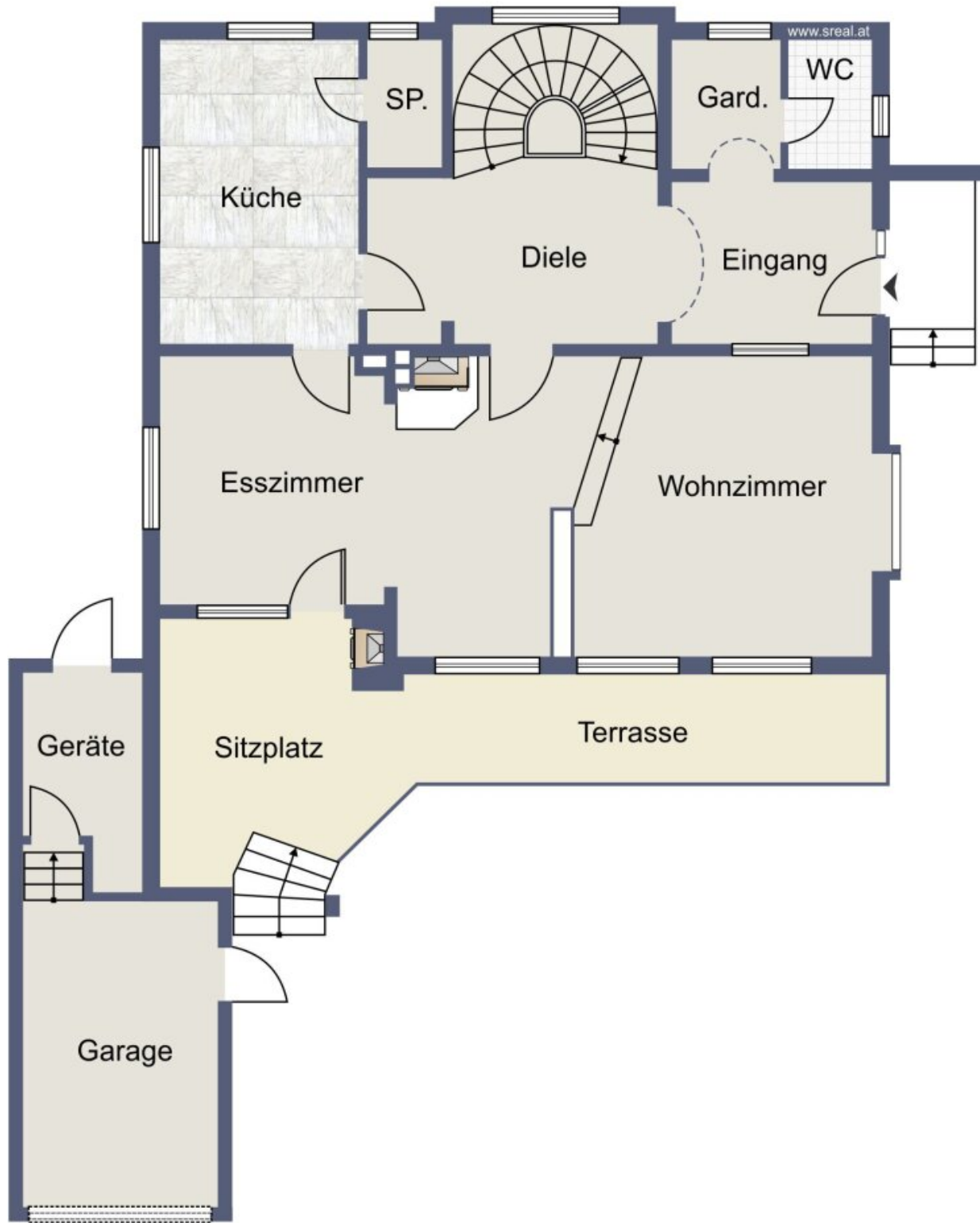
Skizze Erdgeschoss
