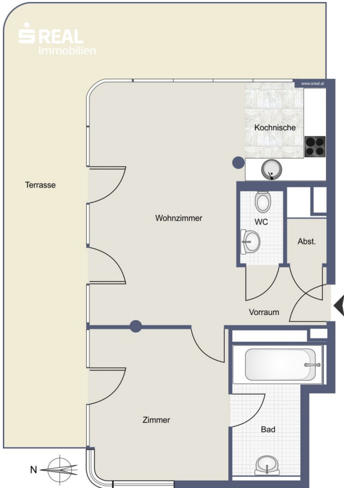
Skizze 19.Obergeschoss
