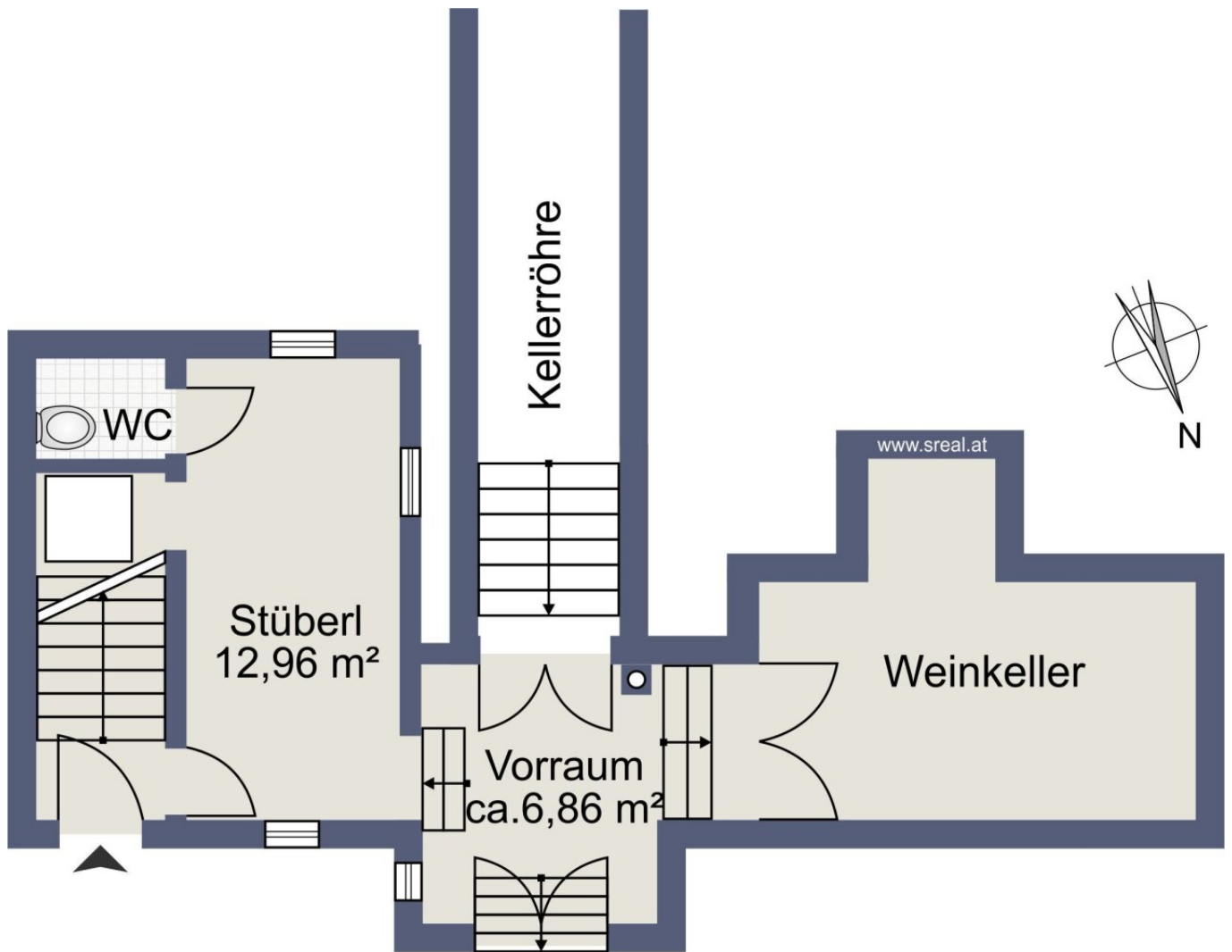
Skizze Kellergeschoss
