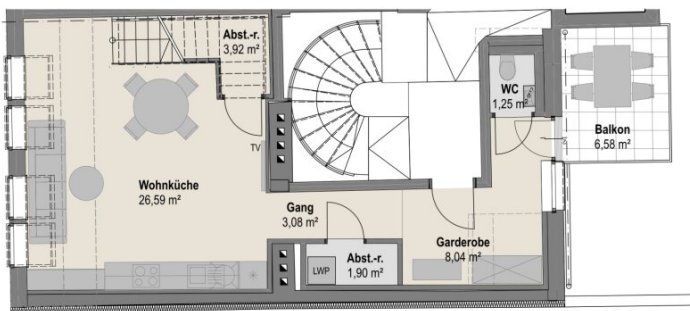
Dachgeschoss 1
