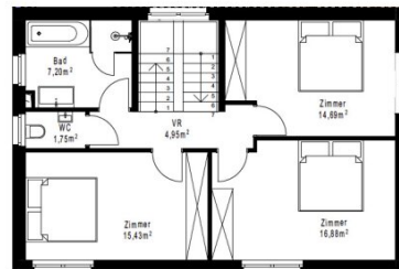
Obergeschoss 1:100
