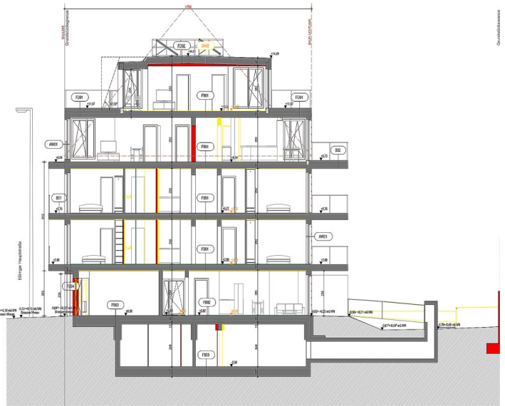
SCHNITT B
