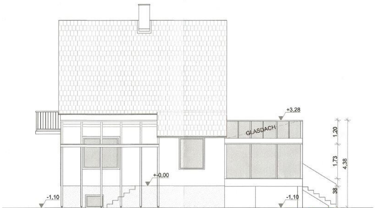
ANSICHT - SÜD
