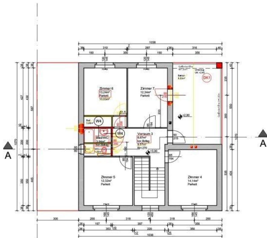
BV 2460 Bruck/L., Dr. Otto Tschadekstraße 38 Obergeschoß M 1:100 17.3.2009
