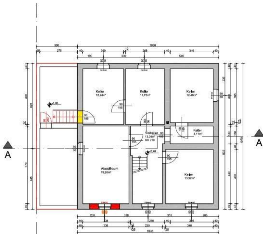
BV 2460 Bruck/L., Dr. Otto Tschadekstraße 38 Kellergeschoß M 1:100 17.3.2009
