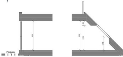
Schnitt 2/70 A
