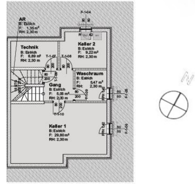
Reihenhausplan | RH 5, Kellergeschoss
