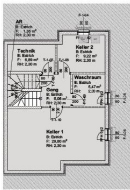
Reihenhausplan | RH 9, Kellergeschoss
