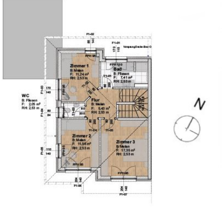
Reihenhausplan RH 11, Obergeschoss
