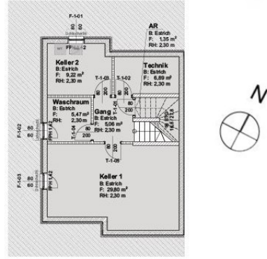
Reihenhausplan RH 11, Kellergeschoss
