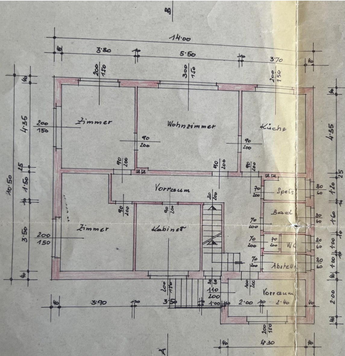
ERDGESCHOSS
