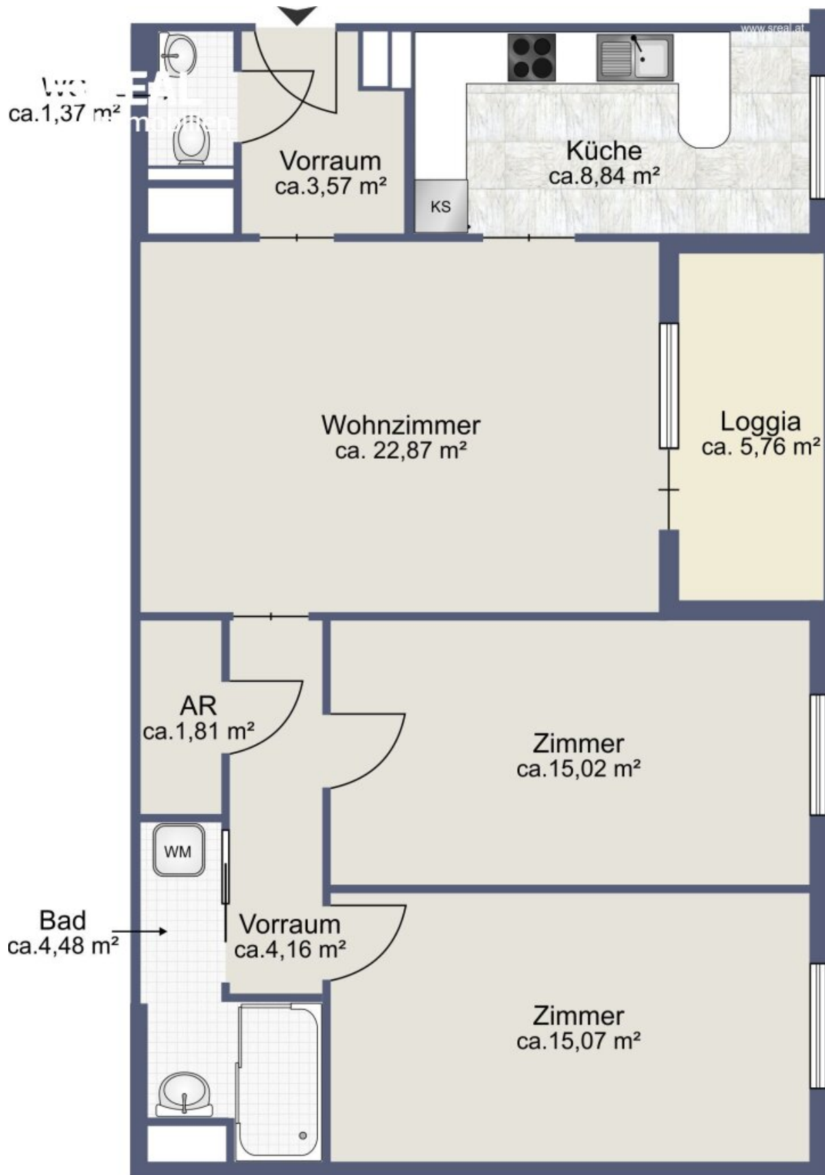
Skizze Obergeschoss
