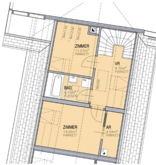
WESTTRAKT GRUNDRISS DACHGESCHOSS TOP 7
