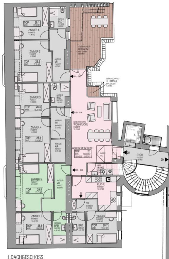
1. DACHGESCHOSS
