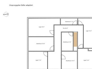
Umgrünungen Keller adaptiert
