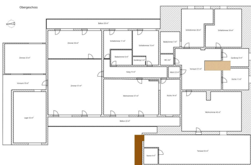
Obergeschoss
