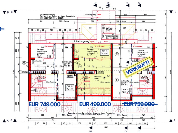
grundriss DG 2
