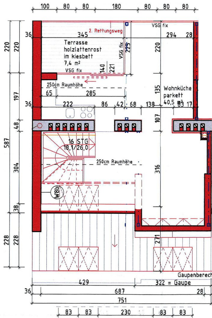
grundriss DG 2
