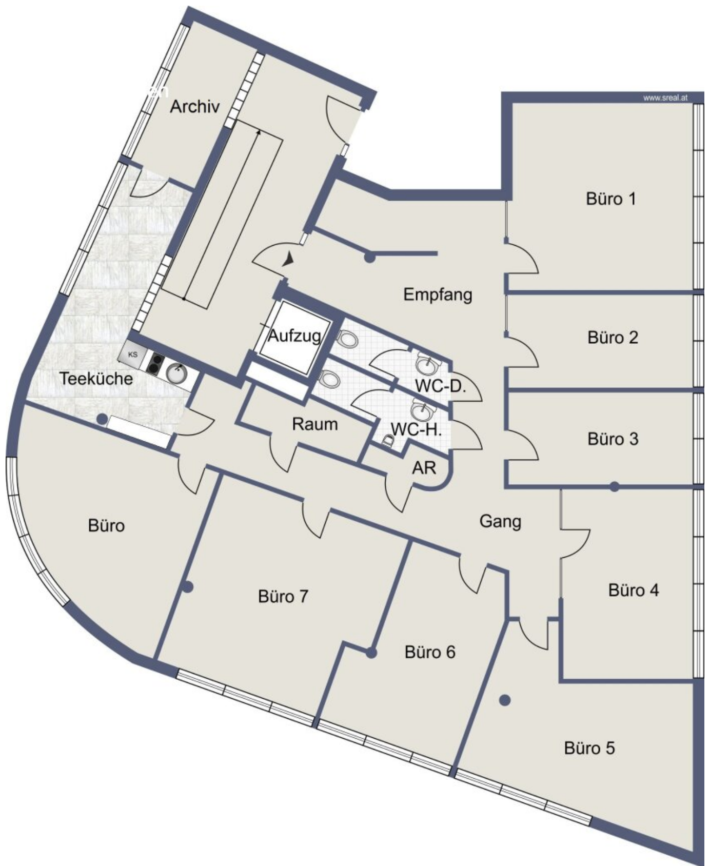
Skizze Obergeschoss 2
