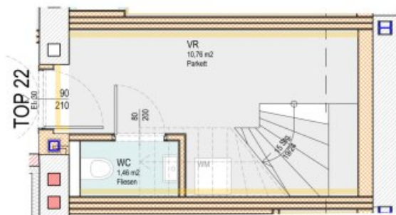
TOP 22 - Grundriss 1.DG
