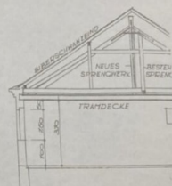
SCHNITT C-D
