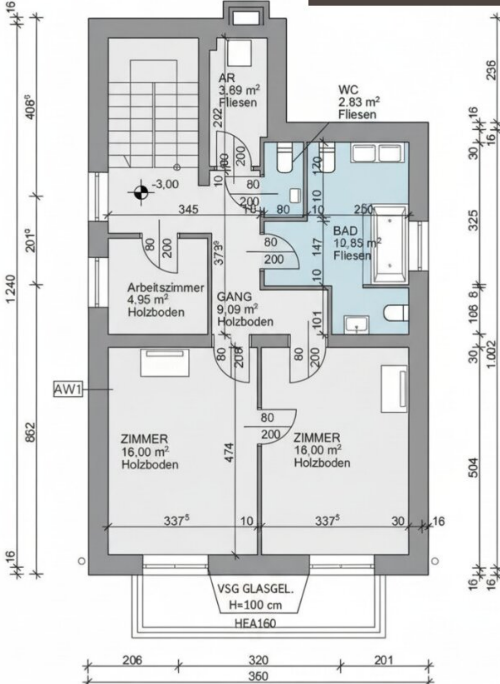
Mittelgeschoss
