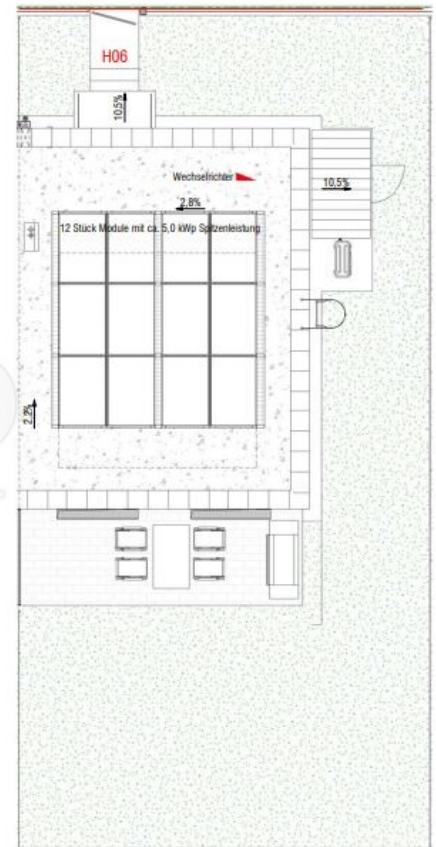
Dachdraufsicht
