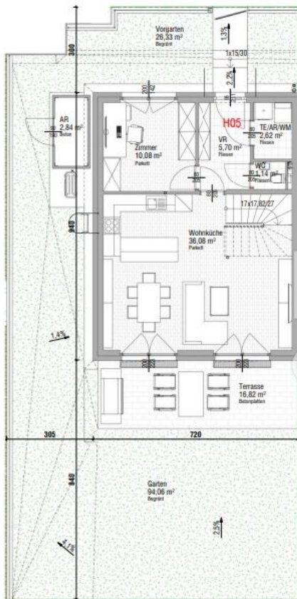
Erdgeschoss
