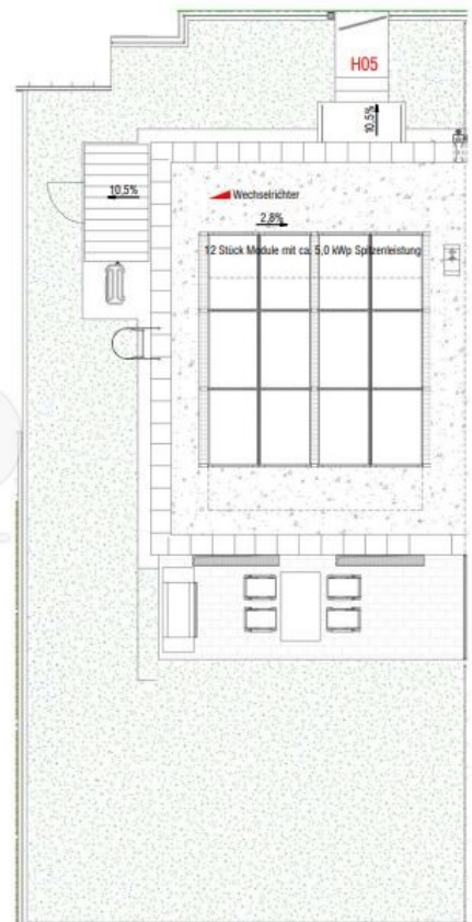
Dachdraufsicht
