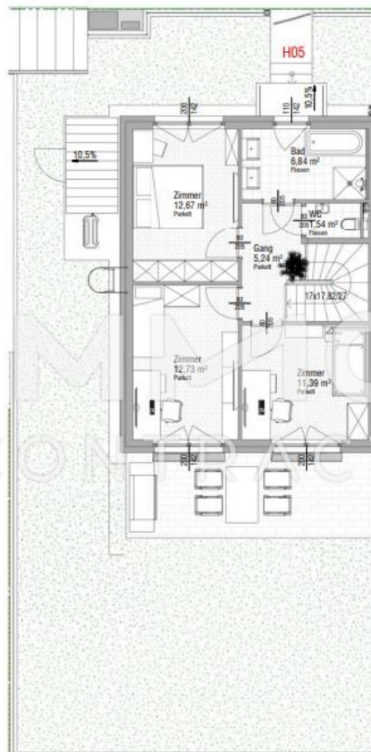
Obergeschoss
