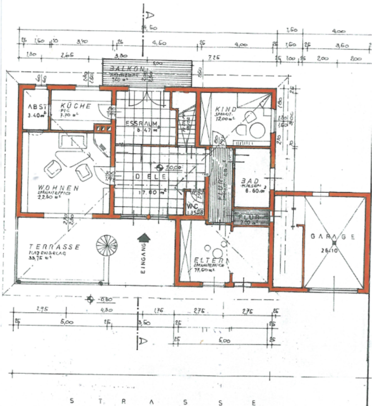
GRUNDRISS ERDGESCHOSS
