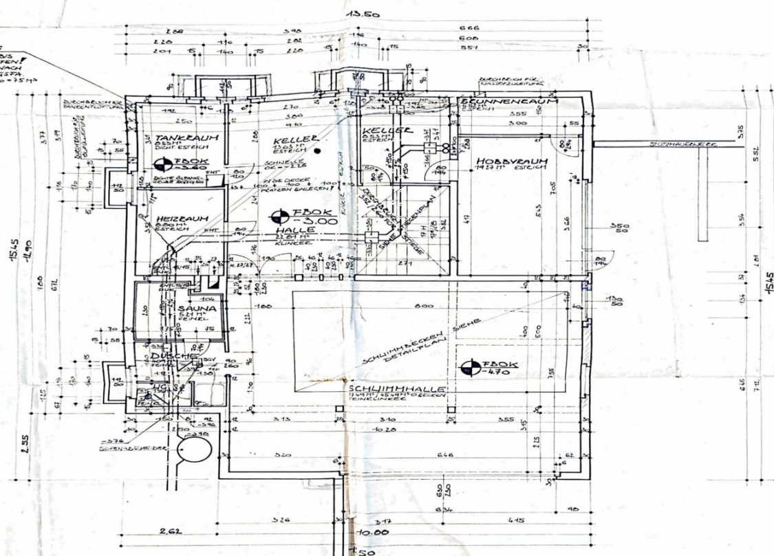
UNTERGESCHOSS M 1:50
