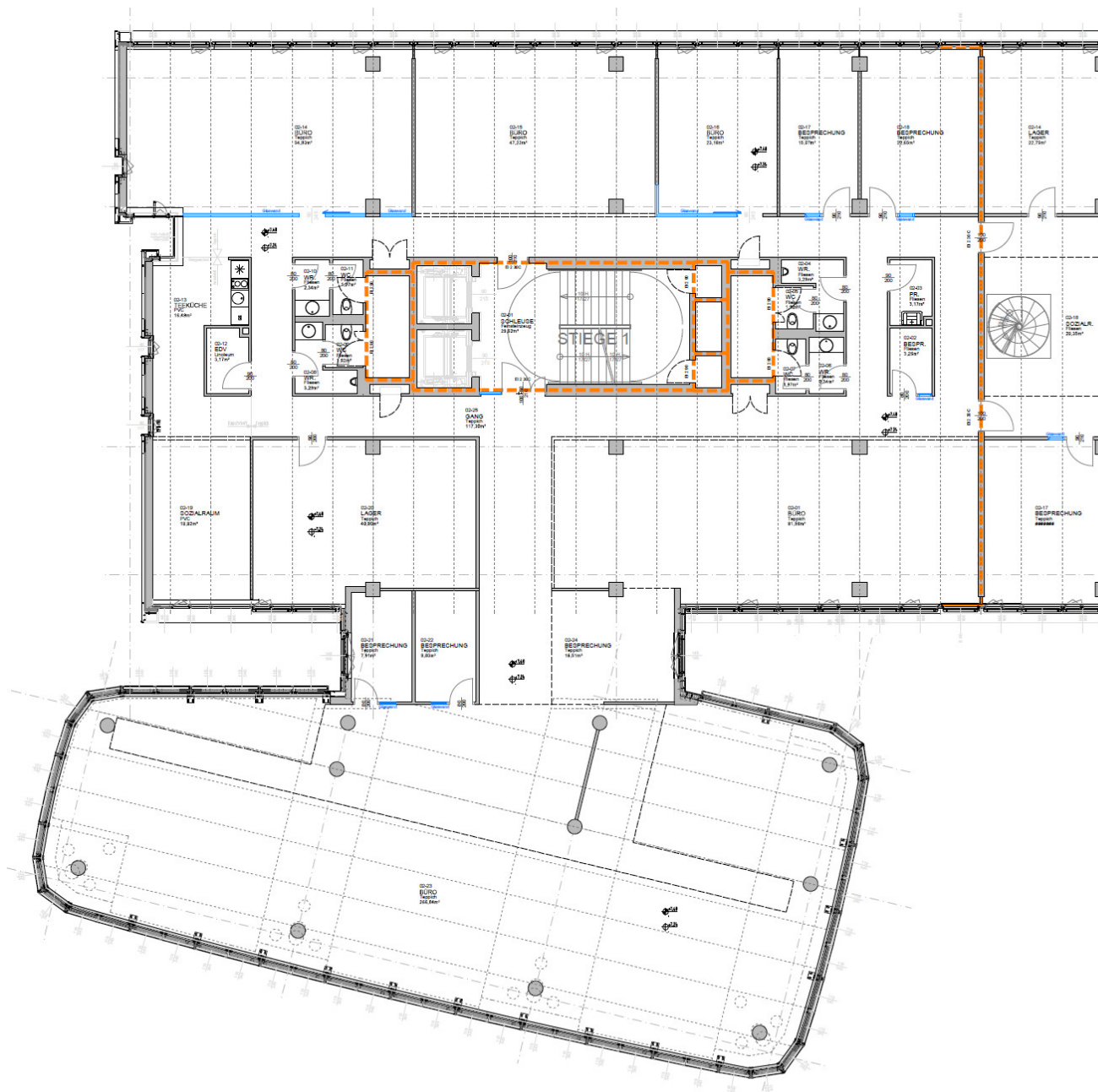
S 2.OBERGESCHOSS
