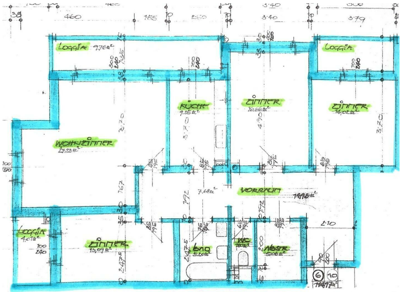
Grundriss.
