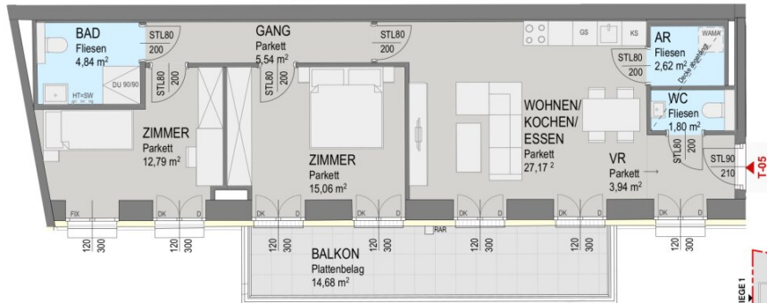
Grundriss 3 OG:
