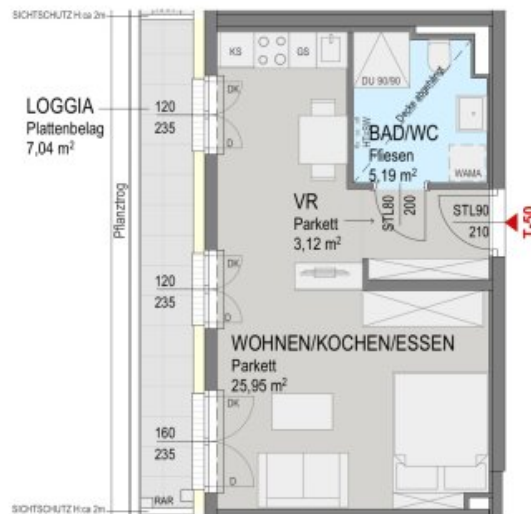
Grundriss 1 DG:
