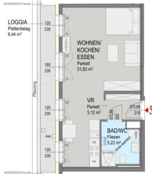
Grundriss 1 DG:
