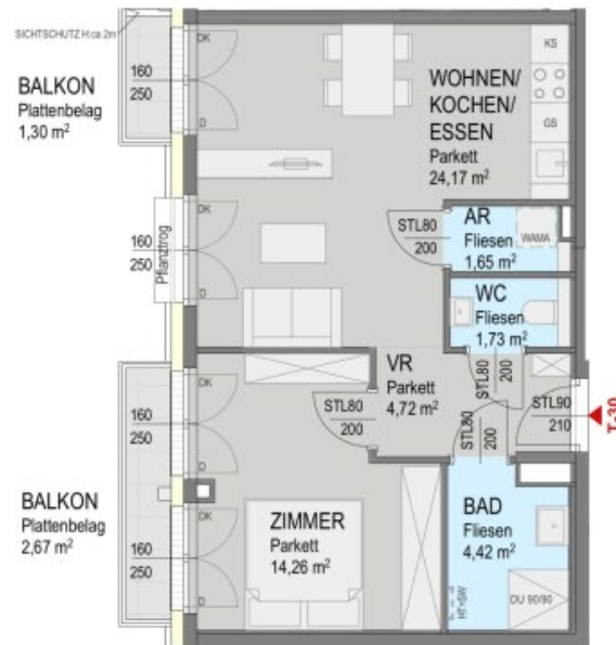
Grundriss 3 OG:
