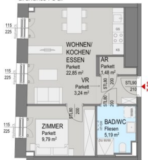
Grundriss 1 OG:
