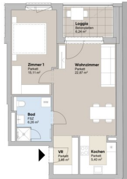
2. Obergeschoß
