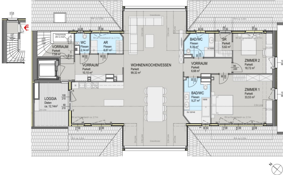
Grundriss Dachgeschoss
