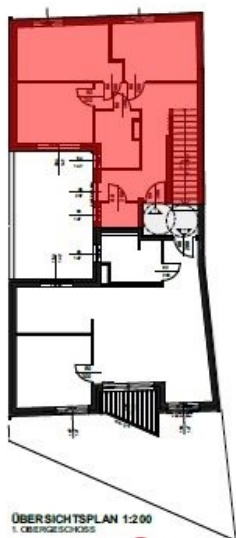
GRUNDRISS 1. OBERGESCHOSS
